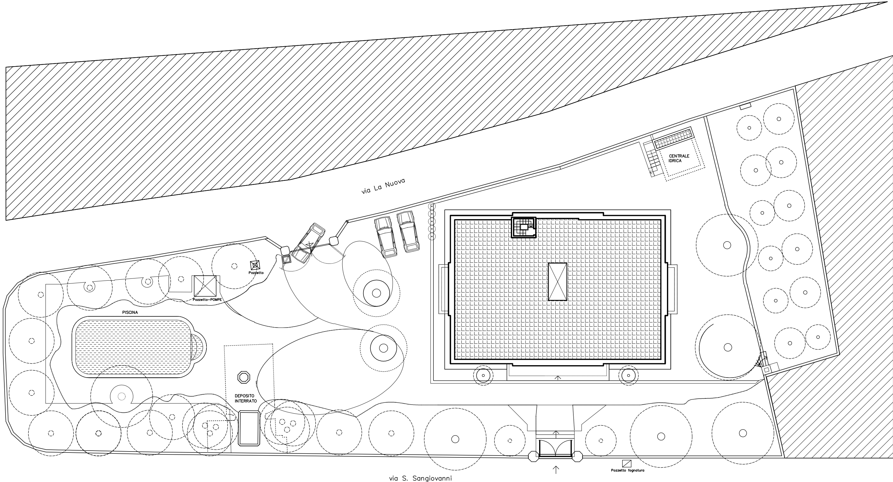
PLANIMETRIA GENERALE Rapp. 1:200
